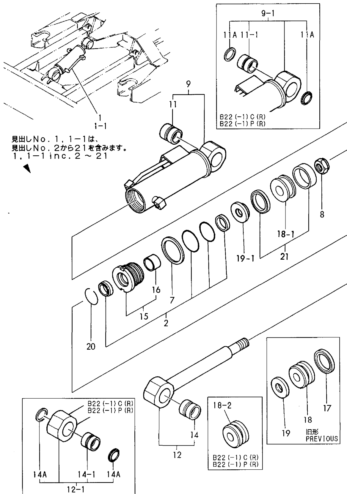
Fig. 37 ブレードシリンダ BLADE CYLINDER
