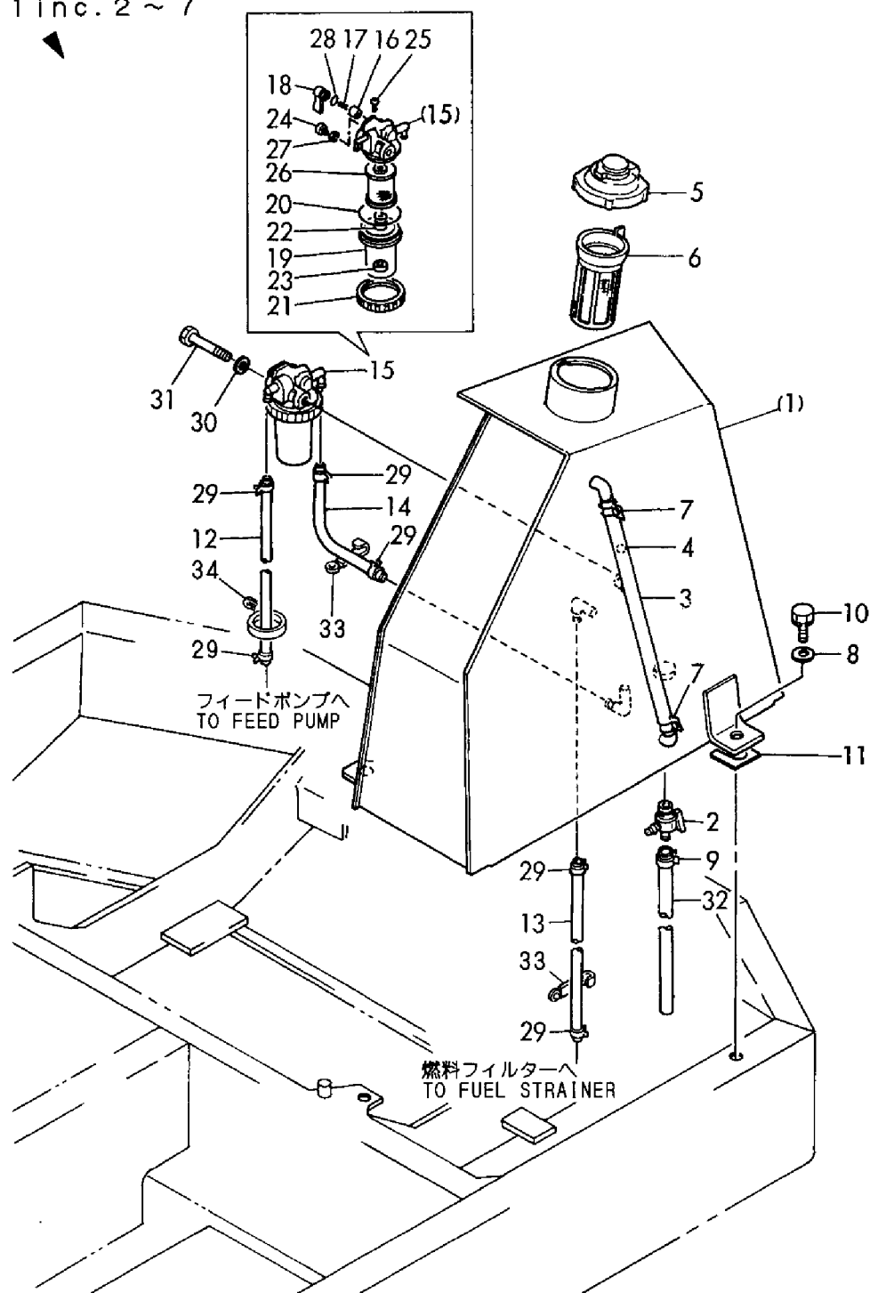
Fig. 7 燃料タンク & 燃料パイプ FUEL TANK & FUEL PIPE
