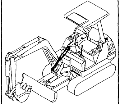
Fig.36 スイングシリンダ (キャノピ) SWING CYLINDER (CANOPY)
