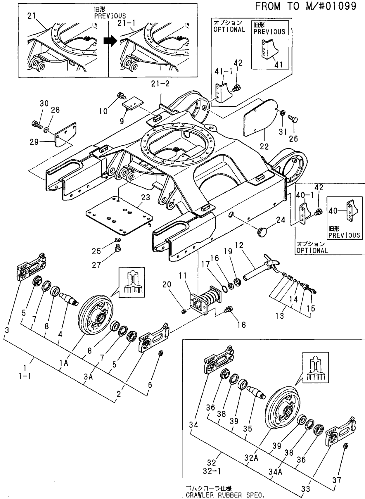
Fig. 17 トラックフレーム&アイドラ (新形) TRACK FRAME & IDLER (NEW)
