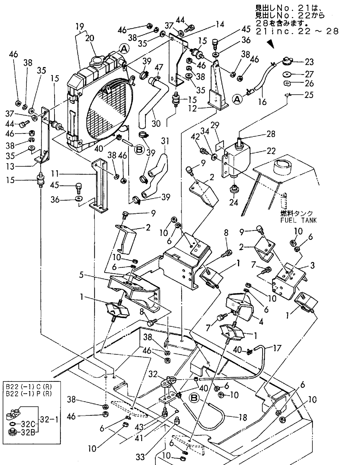
Fig. 6 エンジンマウント & ラジエータ ENGINE MOUNT & RADIATOR
