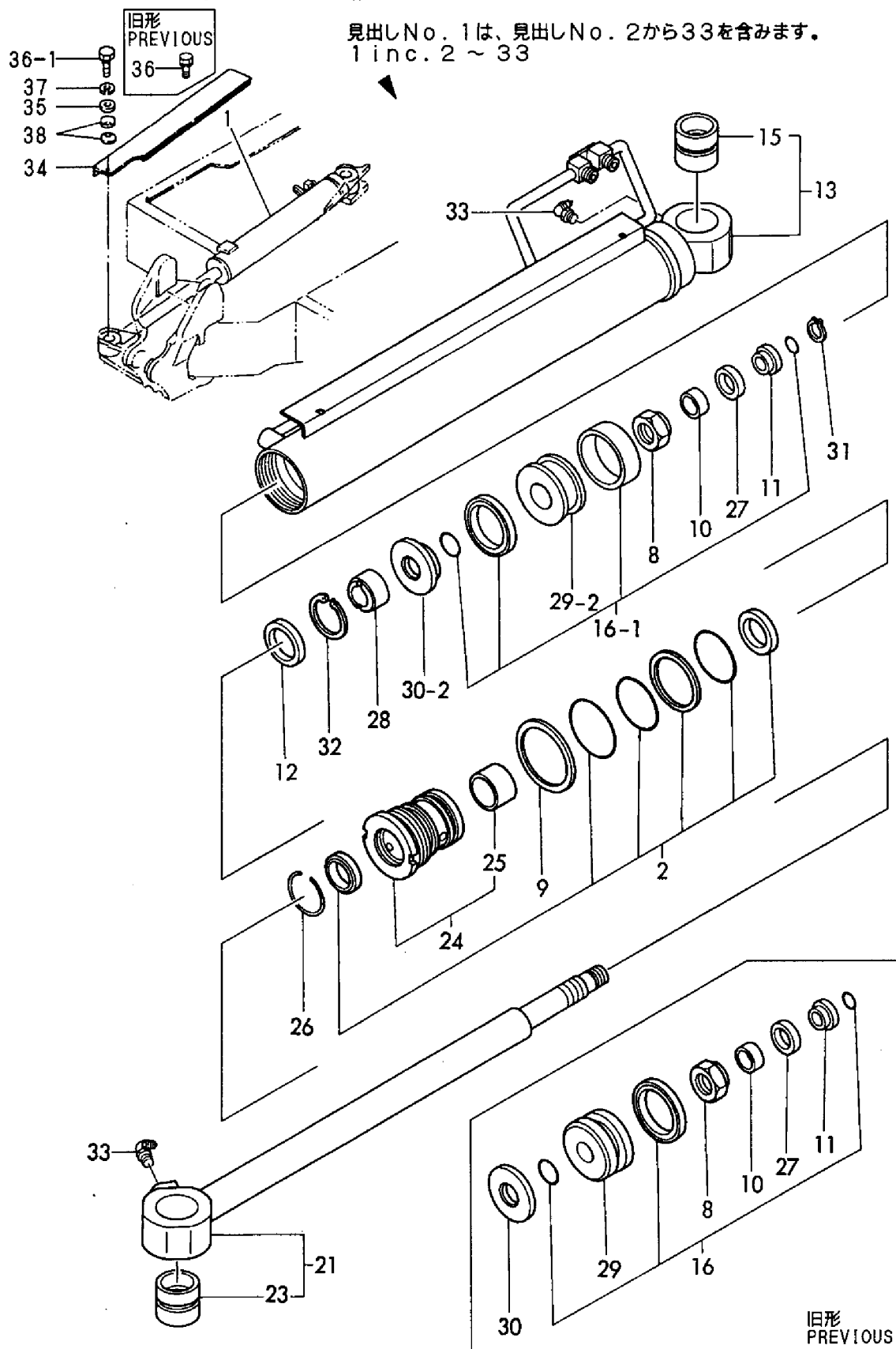
Fig. 36 スイングシリンダ (キャノピ) SWING CYLINDER (CANOPY)
