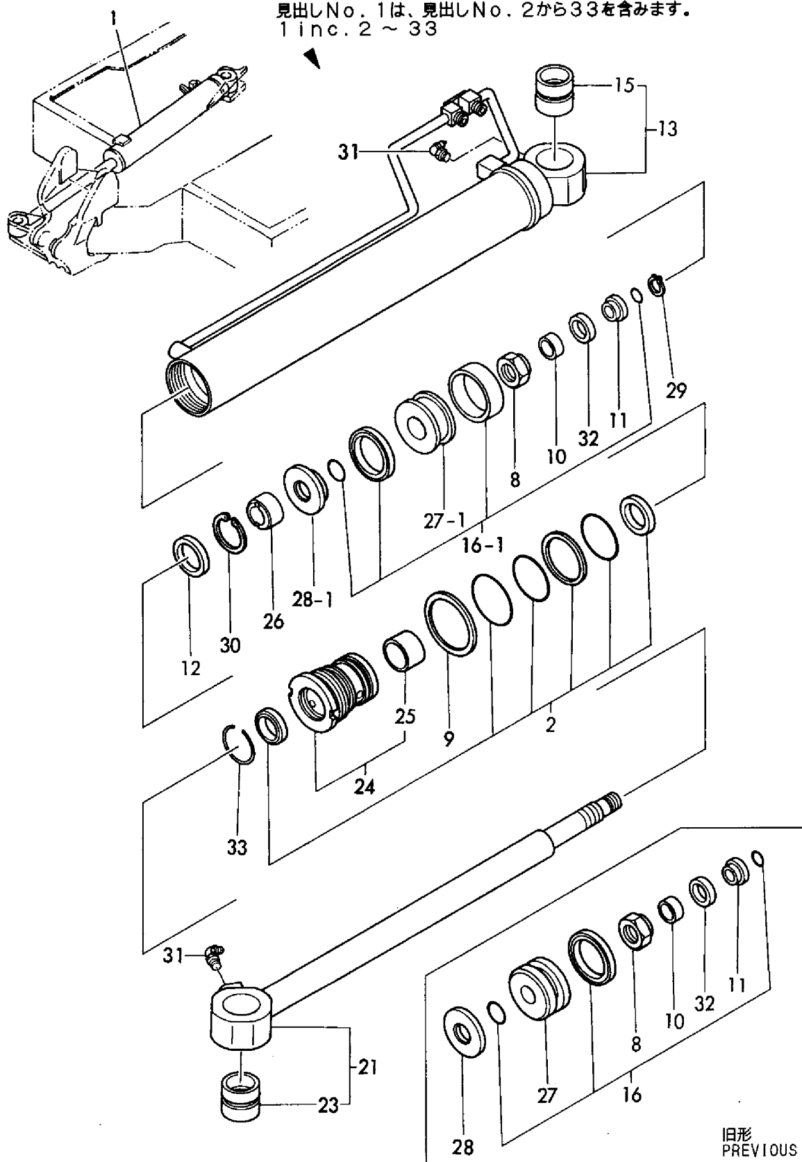
Fig. 35 スイングシリンダ (キャビン) SWING CYLINDER (CABIN)
