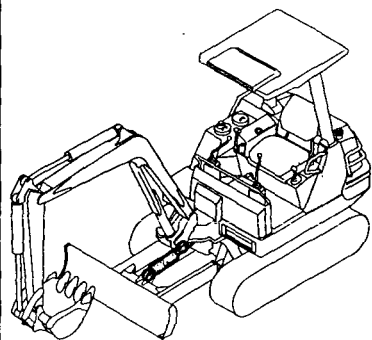
Fig.38 油圧ポンプ&軸継手 HYD.OIL PUMP & JOINT
