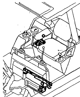
Fig.22 操縦装置 (リンク) (マルチリンク仕様) CONTROL EQUIPMENT (LINK) (MULTI LINK SPEC.)
