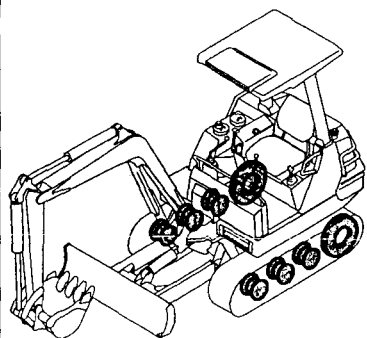
Fig.14 トラックローラ (新形) TRACK ROLLER (NEW)
