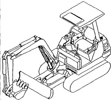
Fig.32 ブームシリンダ (キャノピ) BOOM CYLINDER (CANOPY)
