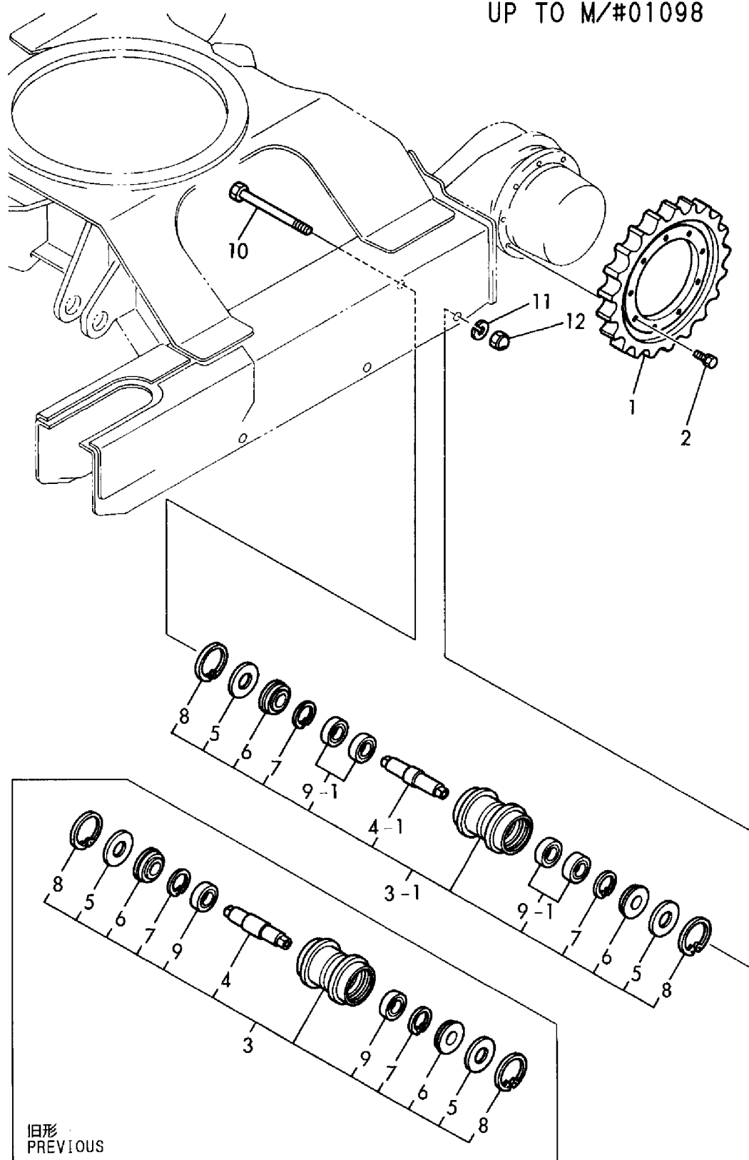
Fig. 12 トラックローラ (旧形) TRACK ROLLER (PREVIOUS)
