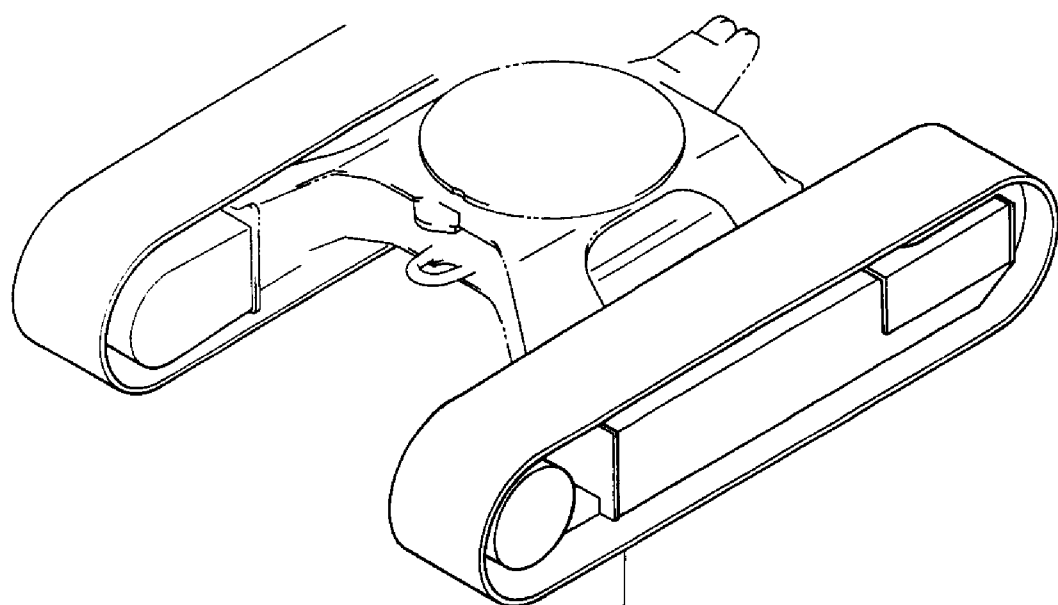
Fig. 60 クローラ (320) (オプション) CRAWLER (320) (OPTIONAL)
