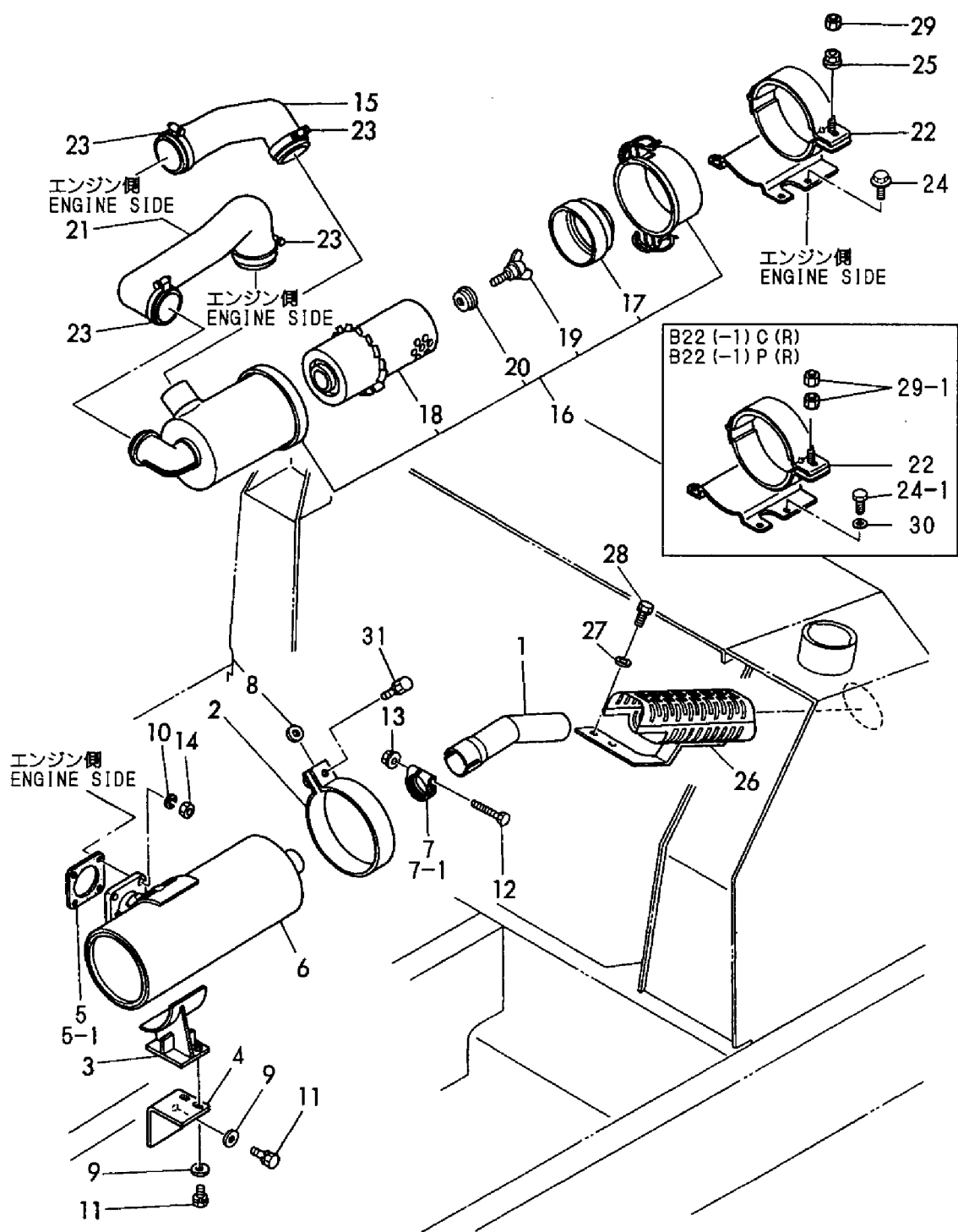
Fig. 4 エアークリーナ&サイレンサ AIR CLEANER & SILENCER
